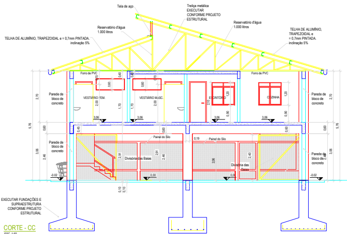
CORTE - CC ESC. 1:50
