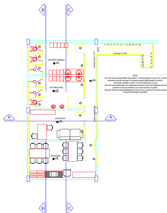
LAYOUT MEZANINO ESC. 1:50
